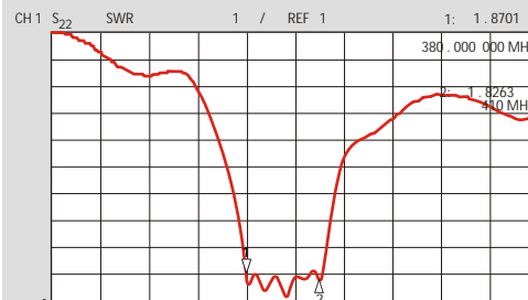
VSWR
