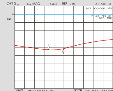
VSWR
