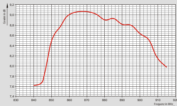
Gewinnverlauf
