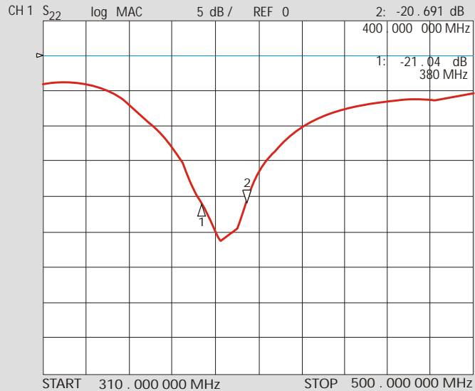
Rückflussdämpfung (Return Loss)
