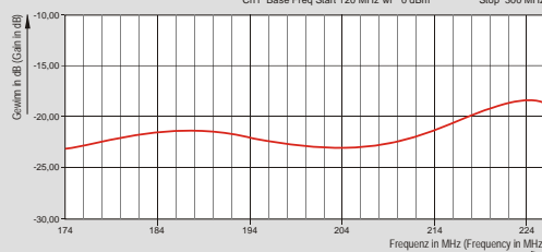
Gewinnverlauf, typisch (Gain progression, typical)
