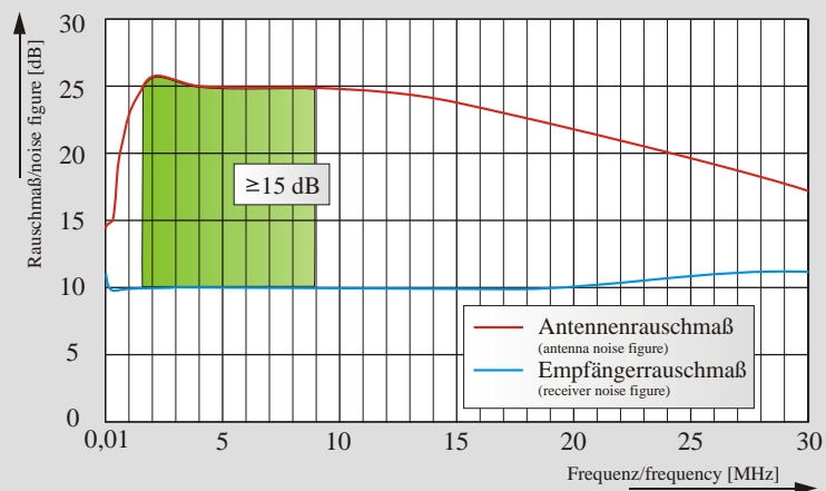
Rauschmaßmessung mit SMV11 Messbandbreite 1,7 kHz, Detektor rms, 50 System (noise figure measurement with SMV 11, bandwidth 1,7 kHz, detector rms, 50 System)
