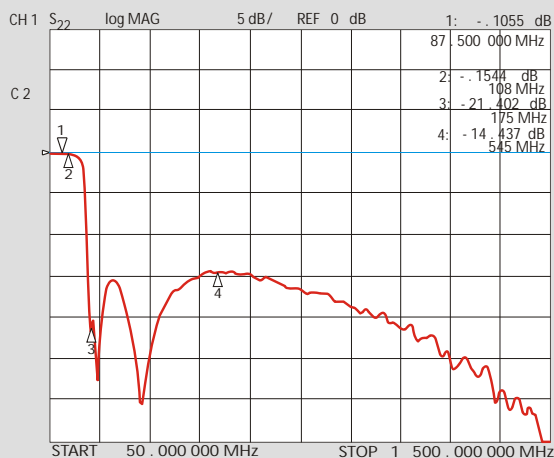
Rückflussdämpfung Port1/Port 2 Return Loss port 1/ port 2
