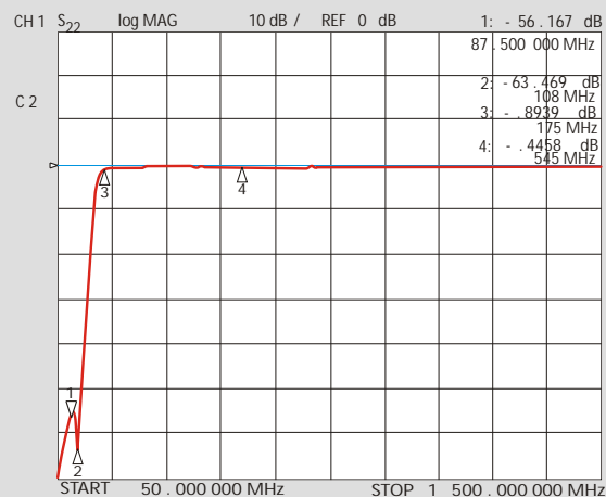
Sperrdämpfung Trap attenuation
